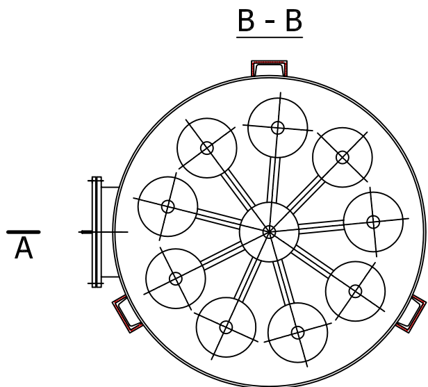
A FILTR CIŚNIENIOWY DN 1.800 PRZEJRÓJ UZBROJENIA I UŁOŻENIA ZŁOŻA FILTRACYJNEGO BEZ SKALI
