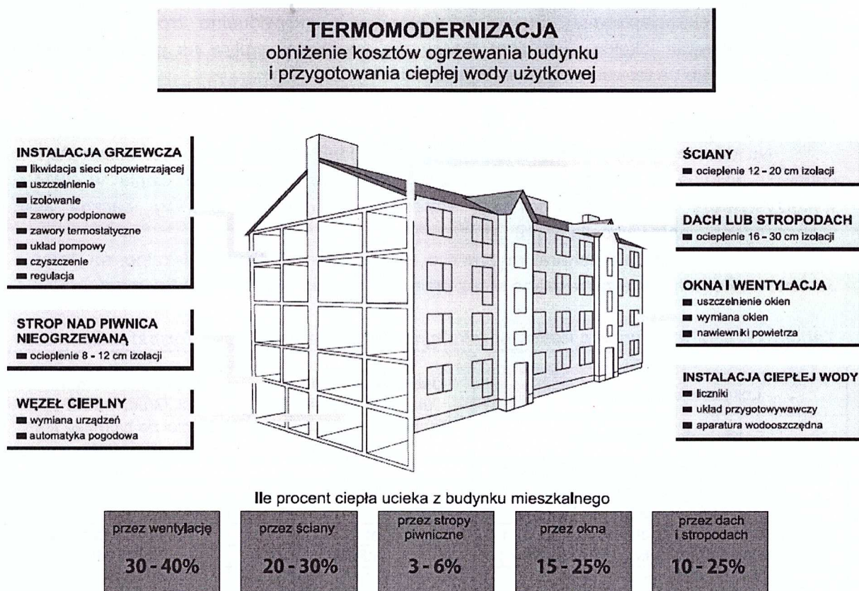
Ryc. 6. Termomodernizacja budynku
